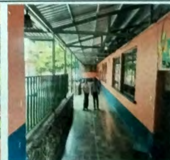
Foto 12: Vista de Modulo de aula, vista corredor, retiro de cielo falso de madera en malas condiciones, cambio de estructura de madera por estructura de metal a base de tijeras y costaneras. Cubierta de asbesto por lamina troquelada cal 26.
